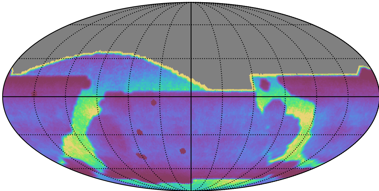
baseline_v3.0_10yrs : DCRprecision
