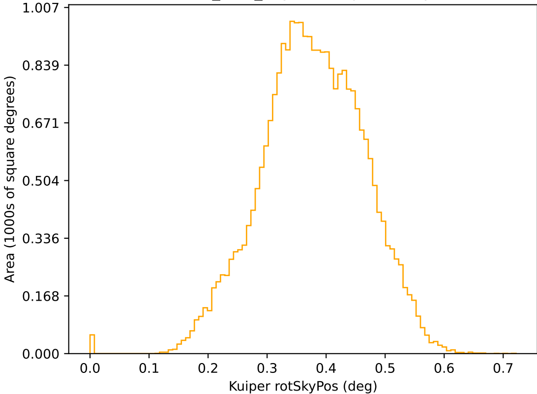
baseline_v3.0_10yrs r: Kuiper rotSkyPos
