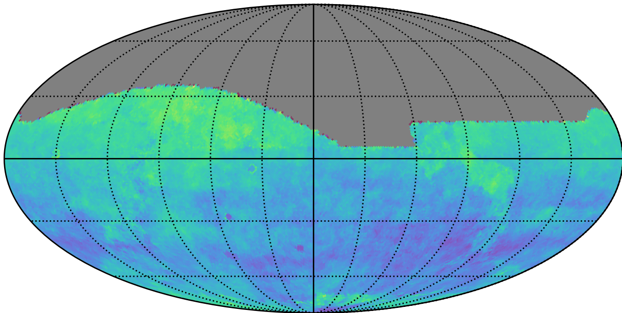
baseline_v3.0_10yrs z: Kuiper rotSkyPos
