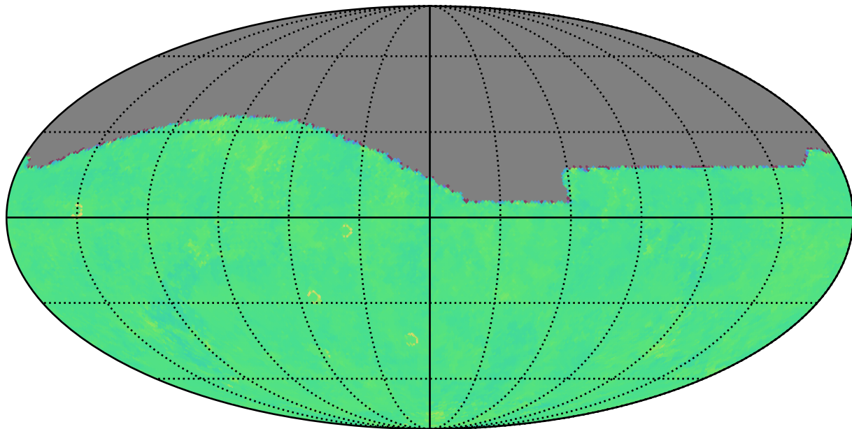
baseline_v3.0_10yrs g: Kuiper rotTelPos
