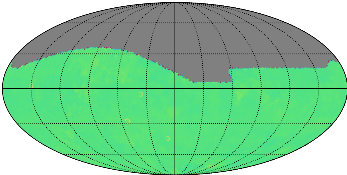
baseline_v3.0_10yrs i: Kuiper rotTelPos
