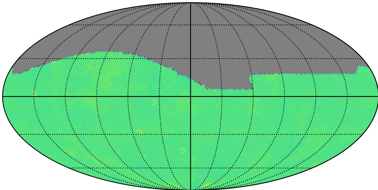
baseline_v3.0_10yrs r: Kuiper rotTelPos
