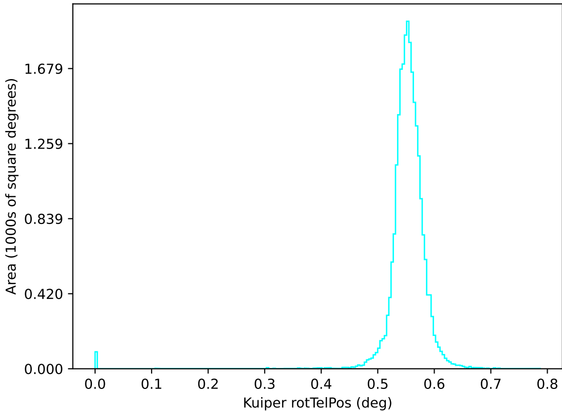
baseline_v3.0_10yrs u: Kuiper rotTelPos
