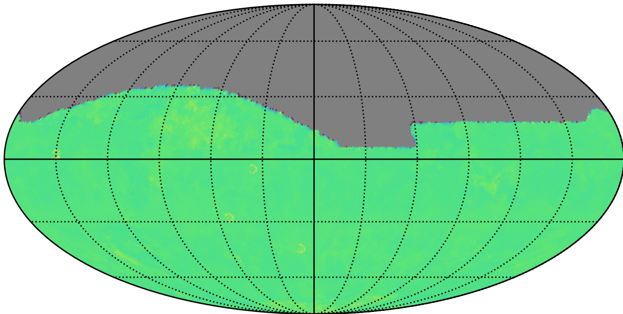
baseline_v3.0_10yrs z: Kuiper rotTelPos
