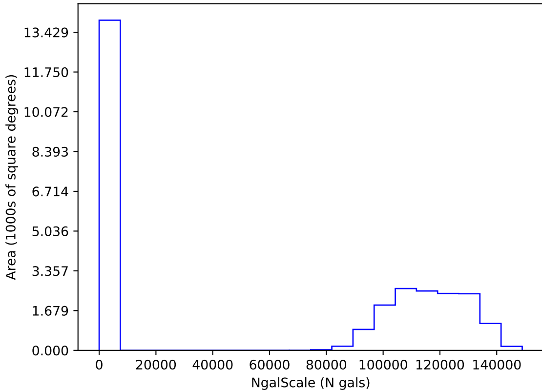
baseline_v3.0_10yrs i: NgalScale
