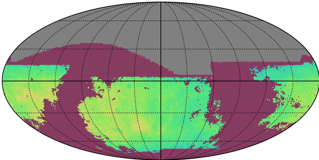
baseline_v3.0_10yrs i: NgalScale
