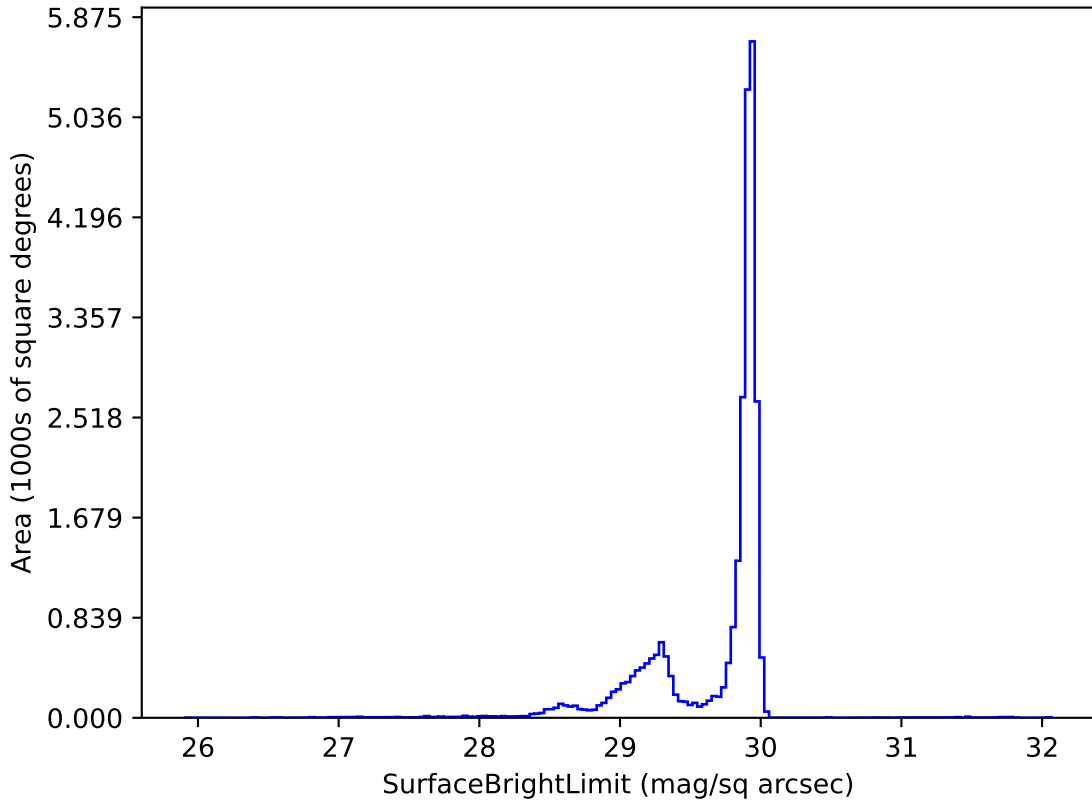
baseline_v3.0_10yrs i: SurfaceBrightLimit
