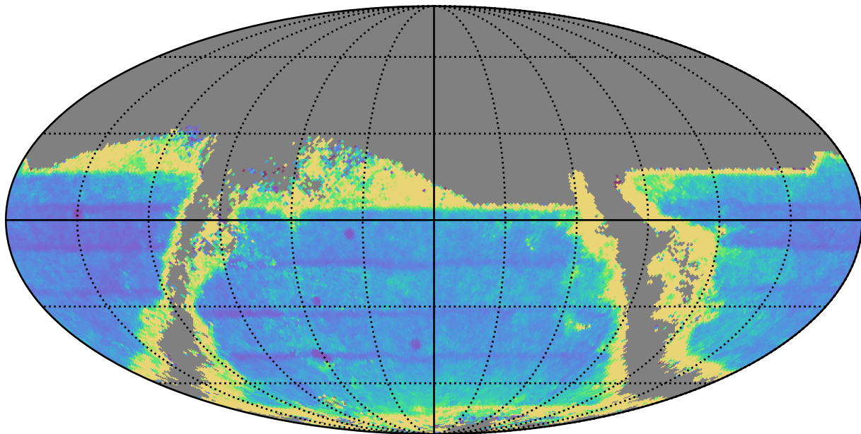
baseline_v3.0_10yrs : TDC_cadence
