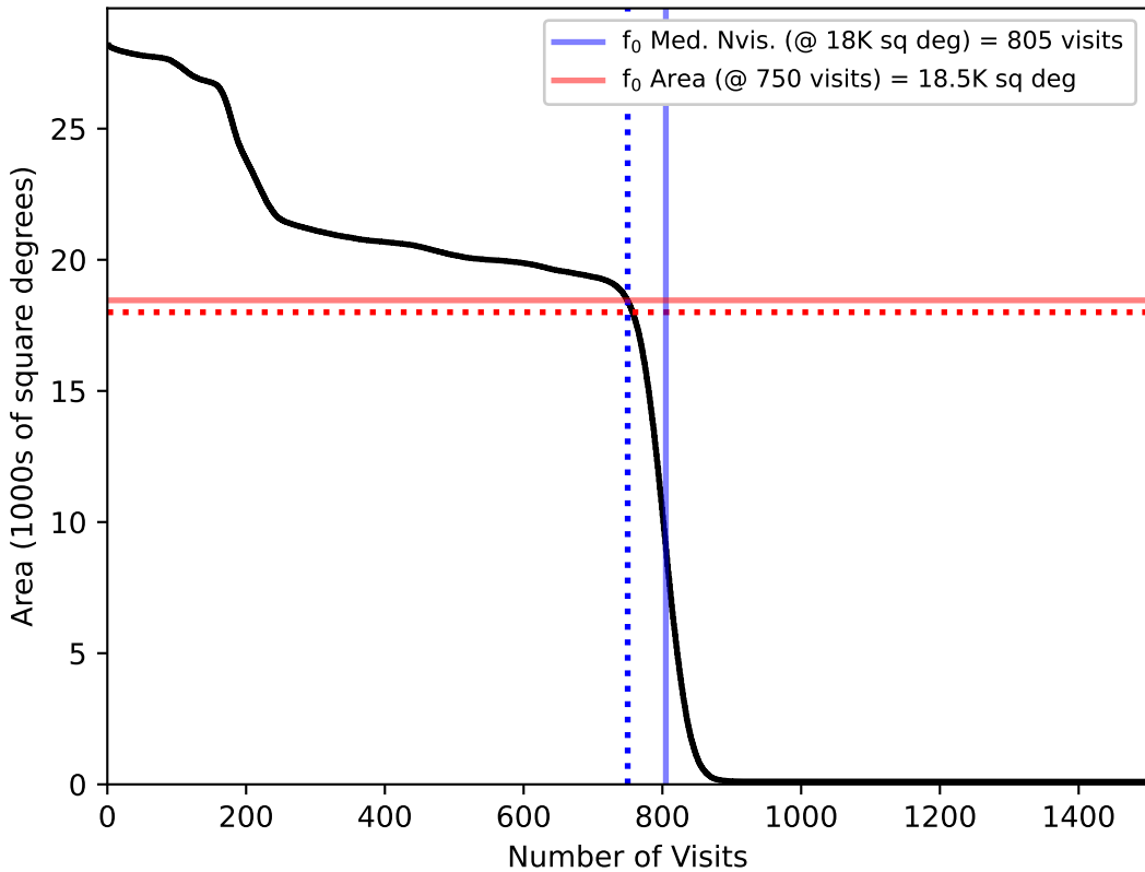
baseline_v3.2_10yrs All sky: f0
