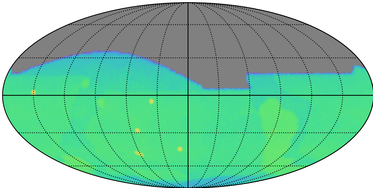
baseline_v3.5_10yrs g: CoaddM5
