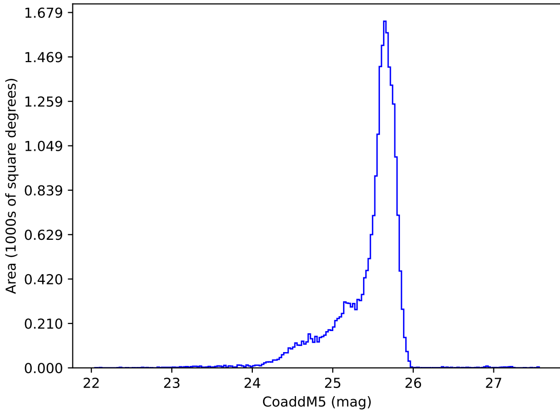
baseline_v3.5_10yrs u: CoaddM5
