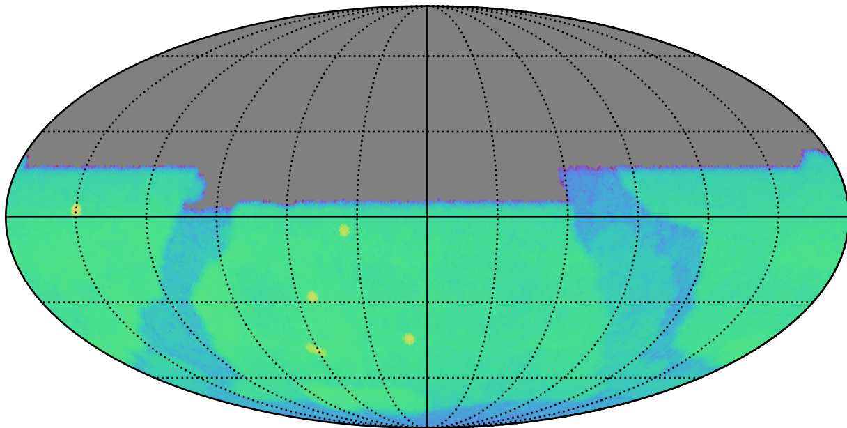
baseline_v3.5_10yrs u: CoaddM5
