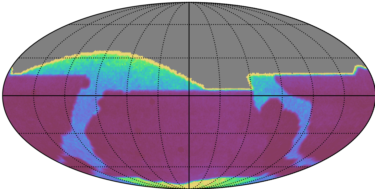
baseline_v3.5_10yrs : properMotion
