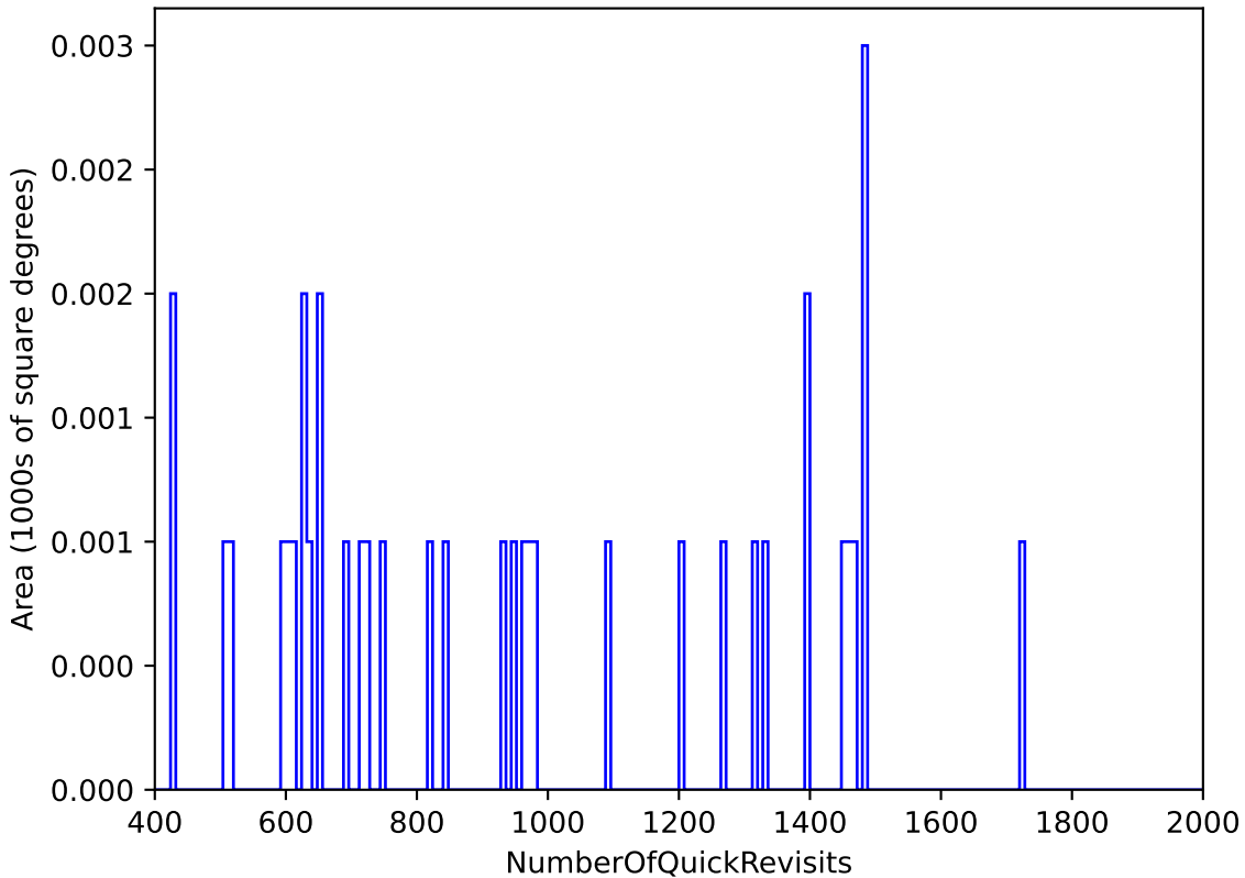
baseline_v3.6_10yrs : NumberOfQuickRevisits
