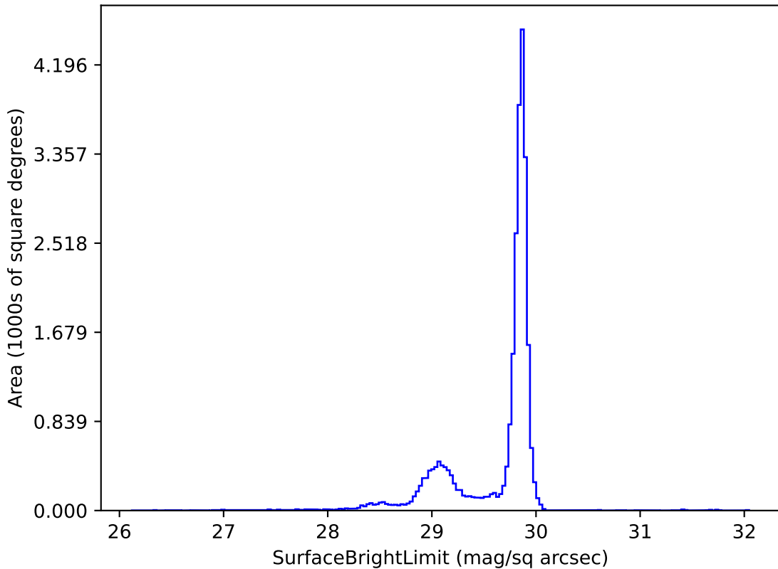
baseline_v3.6_10yrs i: SurfaceBrightLimit
