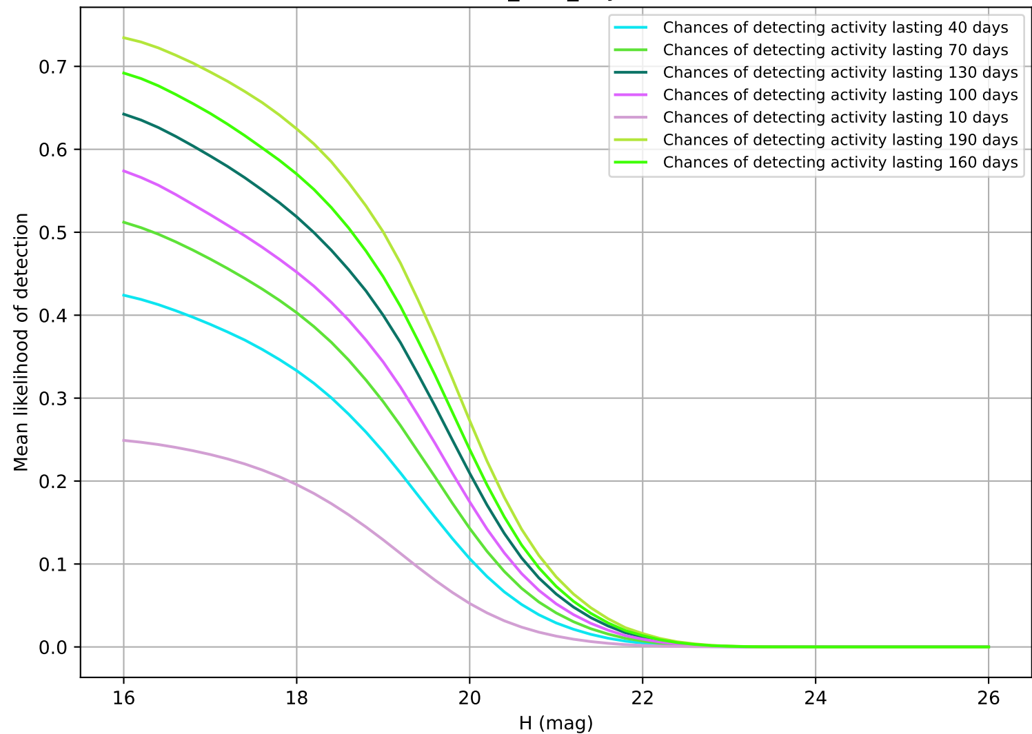
baseline_v3.6_10yrs MBA
