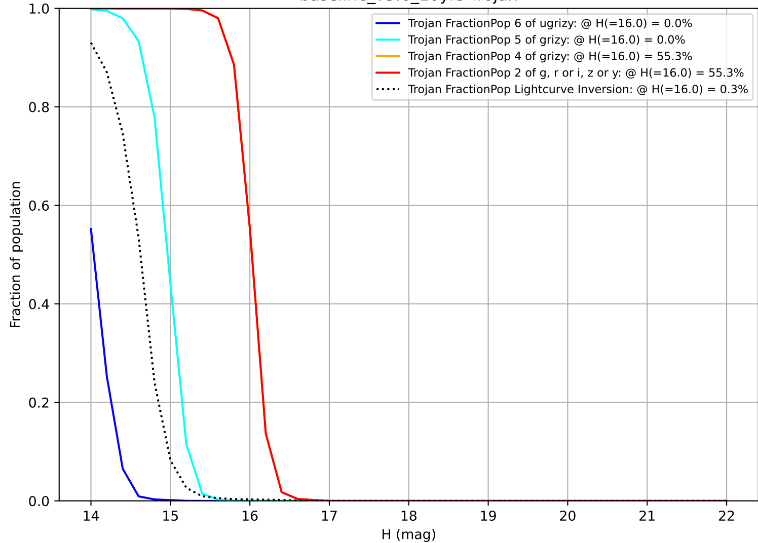
baseline_v3.6_10yrs Trojan
