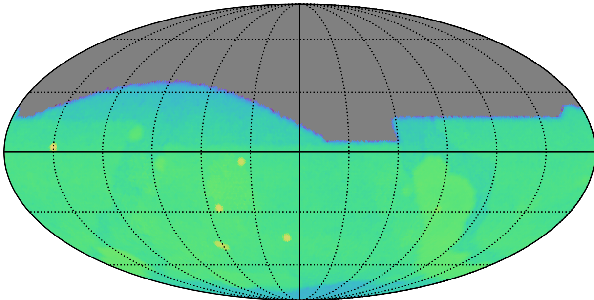
baseline_v4.0_10yrs g: CoaddM5
