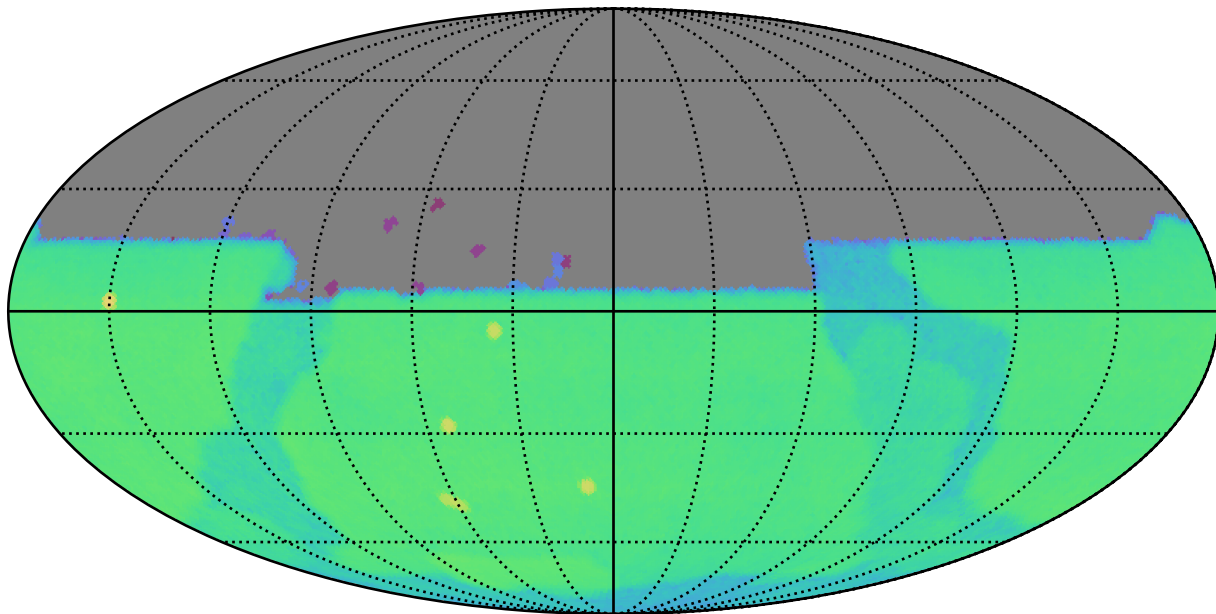
baseline_v4.0_10yrs u: CoaddM5
