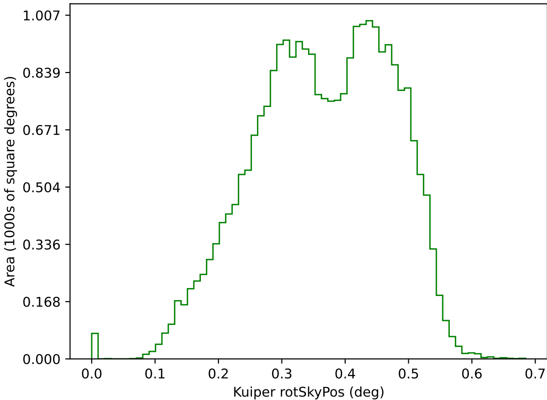
baseline_v4.0_10yrs g: Kuiper rotSkyPos
