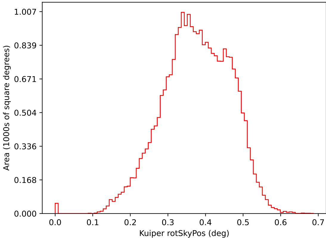
baseline_v4.0_10yrs i: Kuiper rotSkyPos
