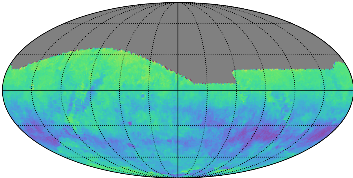
baseline_v4.0_10yrs i: Kuiper rotSkyPos
