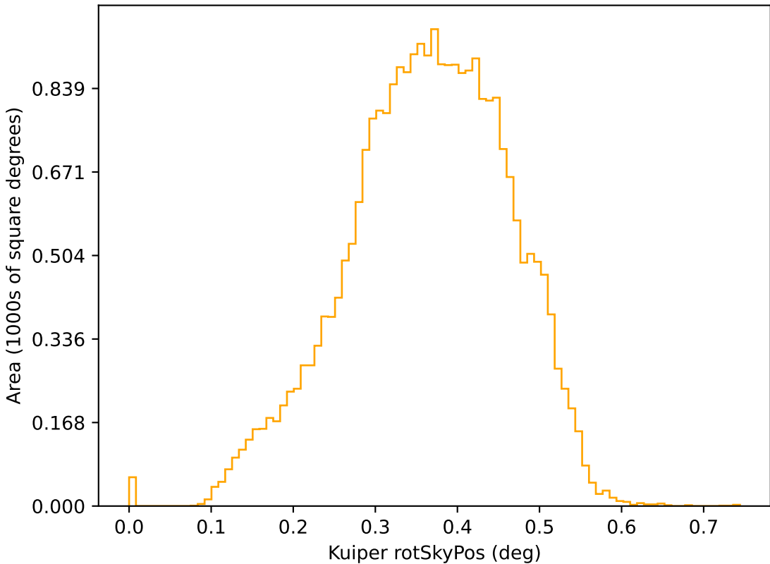
baseline_v4.0_10yrs r: Kuiper rotSkyPos
