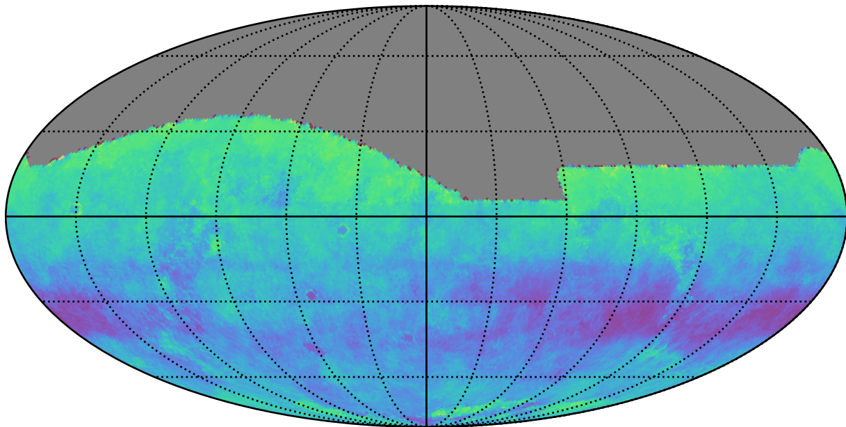
baseline_v4.0_10yrs r: Kuiper rotSkyPos
