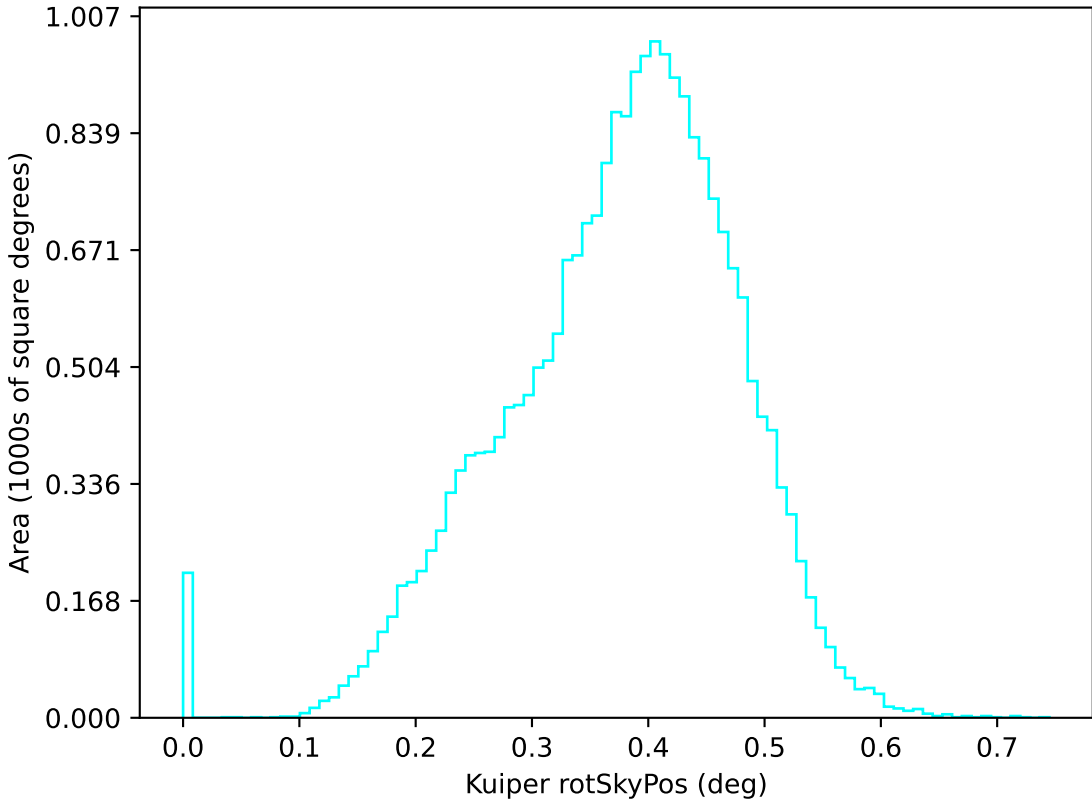
baseline_v4.0_10yrs u: Kuiper rotSkyPos
