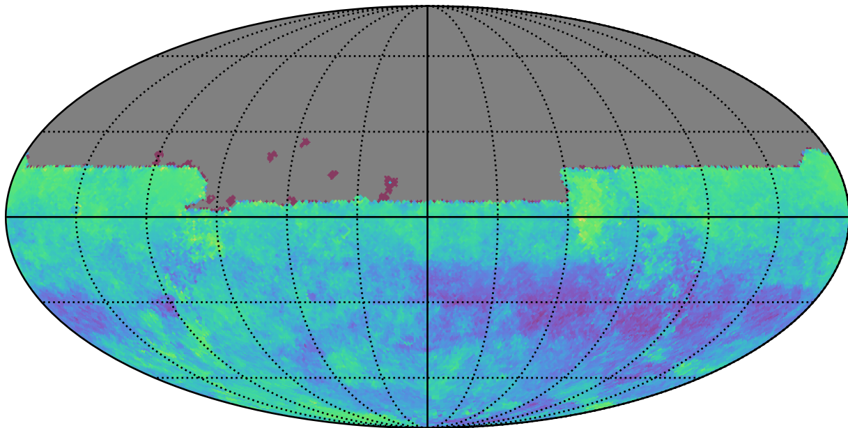
baseline_v4.0_10yrs u: Kuiper rotSkyPos
