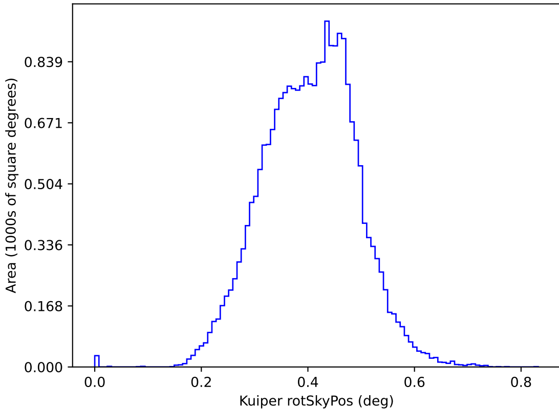
baseline_v4.0_10yrs y: Kuiper rotSkyPos
