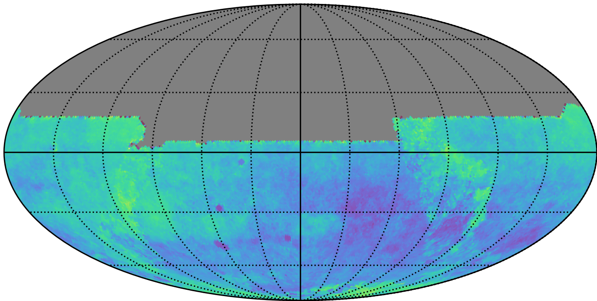
baseline_v4.0_10yrs y: Kuiper rotSkyPos
