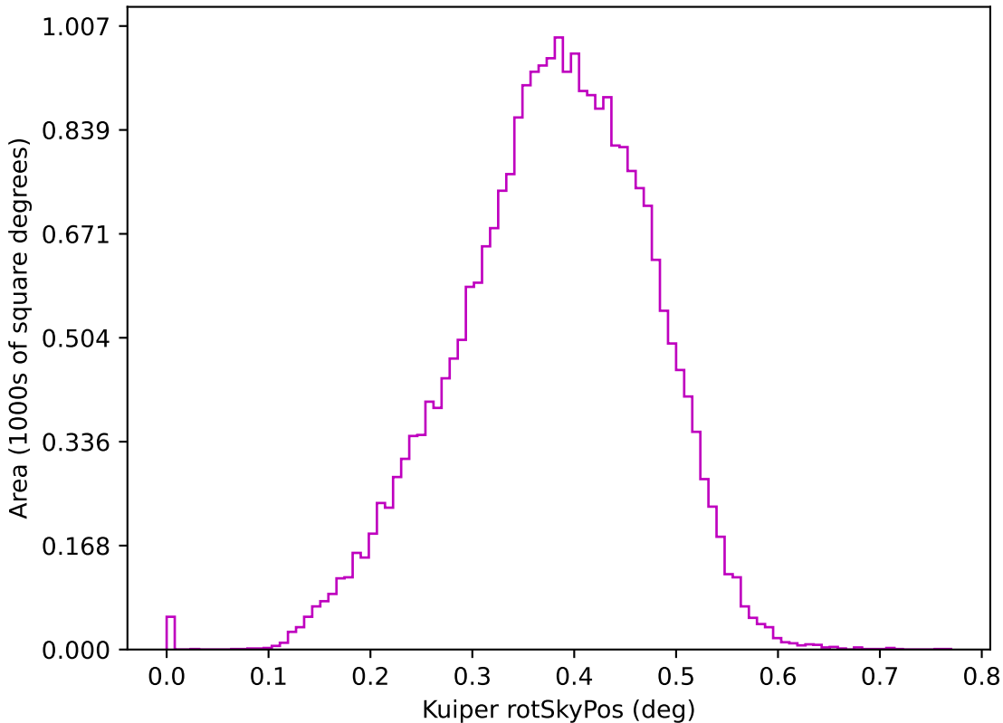
baseline_v4.0_10yrs z: Kuiper rotSkyPos
