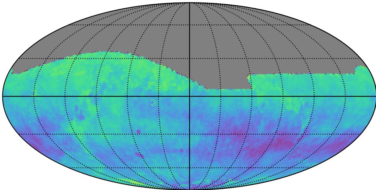
baseline_v4.0_10yrs z: Kuiper rotSkyPos
