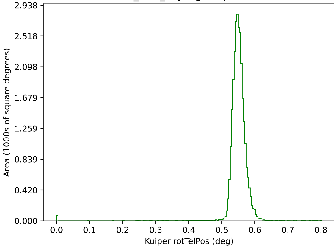
baseline_v4.0_10yrs g: Kuiper rotTelPos
