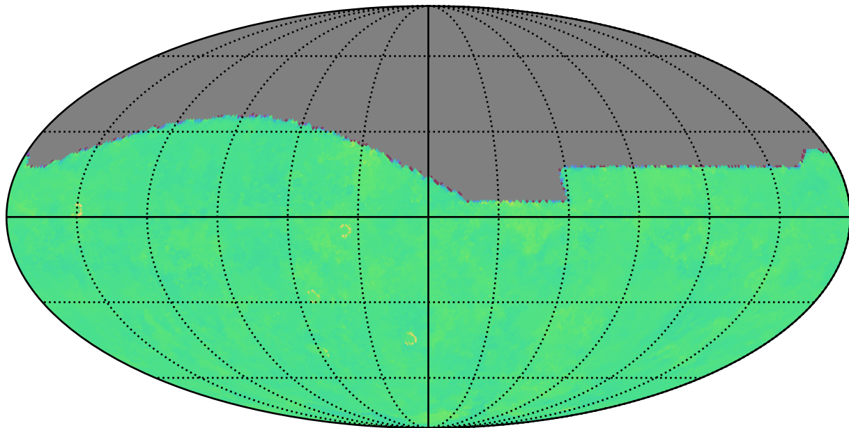
baseline_v4.0_10yrs g: Kuiper rotTelPos
