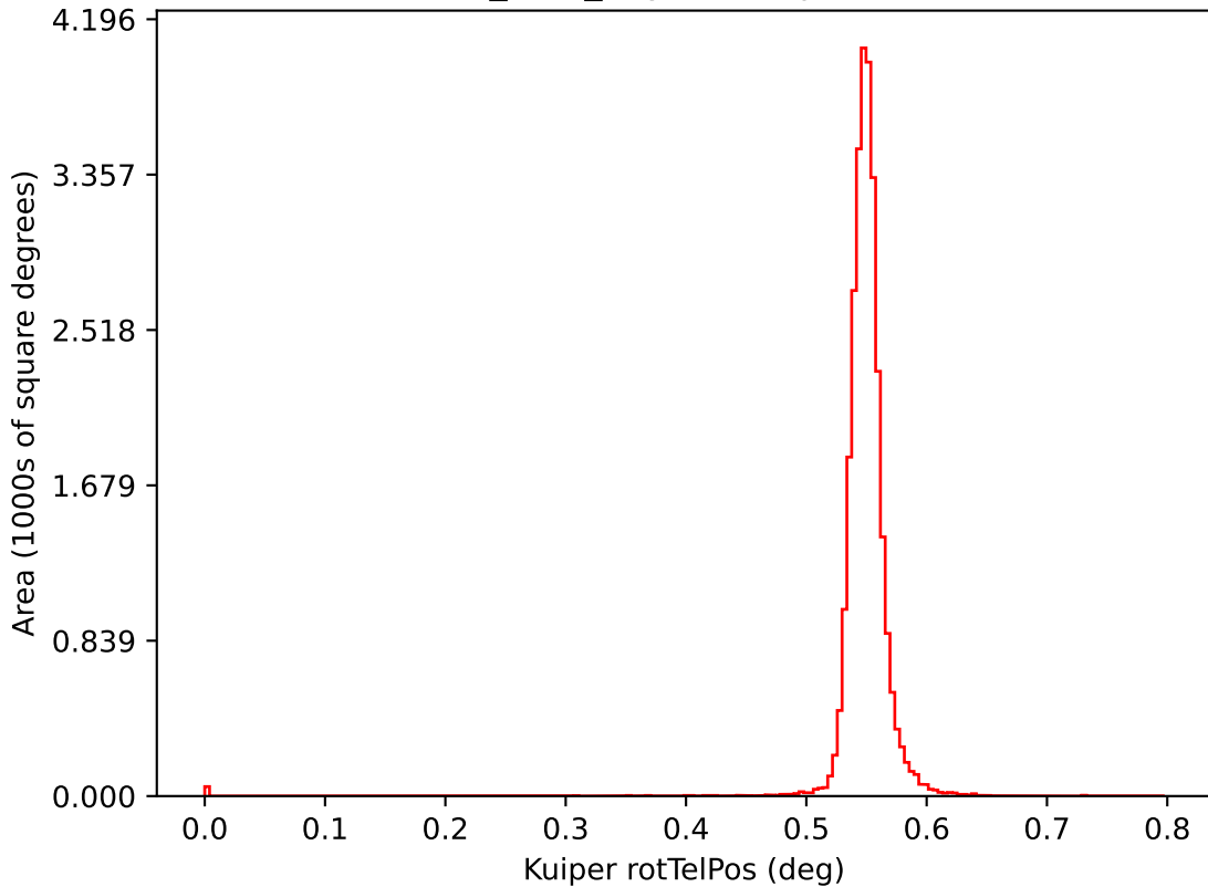
baseline_v4.0_10yrs i: Kuiper rotTelPos
