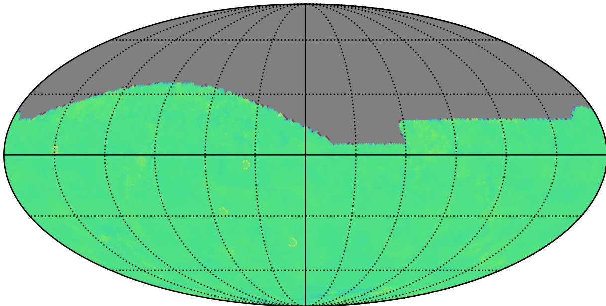
baseline_v4.0_10yrs i: Kuiper rotTelPos
