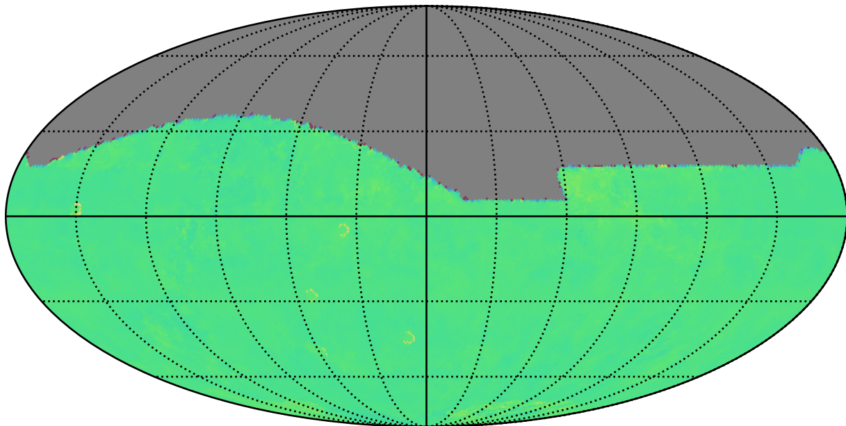
baseline_v4.0_10yrs r: Kuiper rotTelPos
