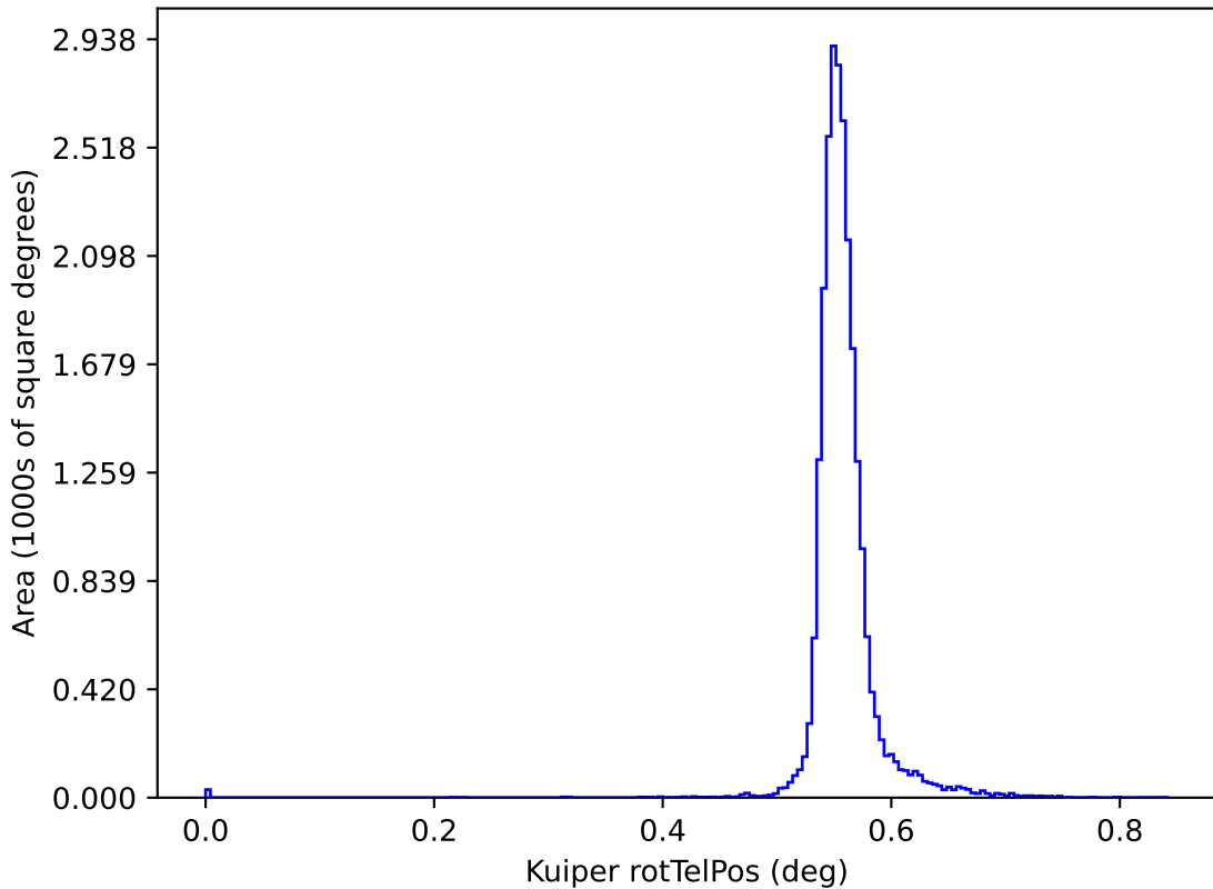
baseline_v4.0_10yrs y: Kuiper rotTelPos
