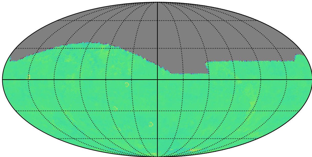
baseline_v4.0_10yrs z: Kuiper rotTelPos
