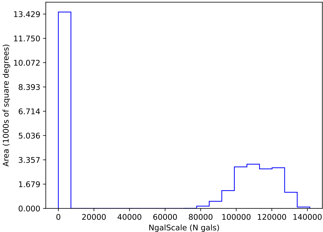
baseline_v4.0_10yrs i: NgalScale
