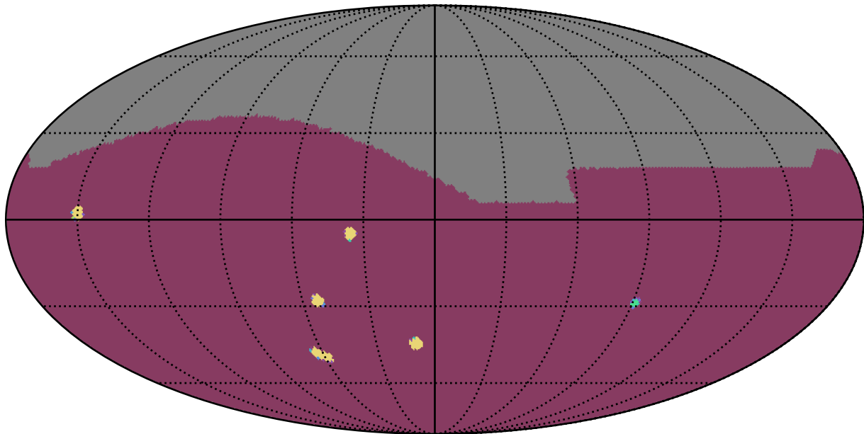
baseline_v4.0_10yrs : NumberOfQuickRevisits
