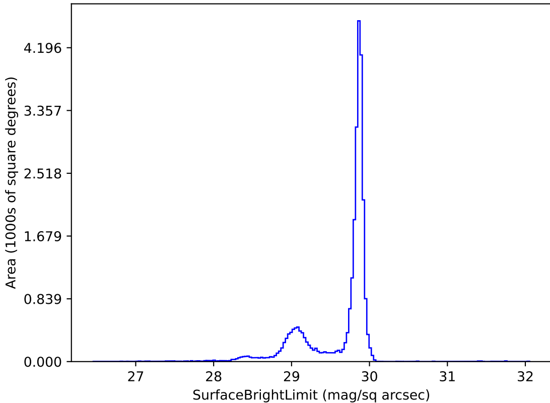
baseline_v4.0_10yrs i: SurfaceBrightLimit
