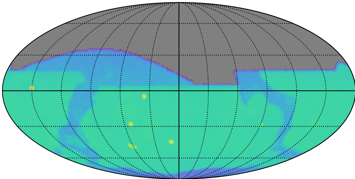
baseline_v4.0_10yrs i: SurfaceBrightLimit
