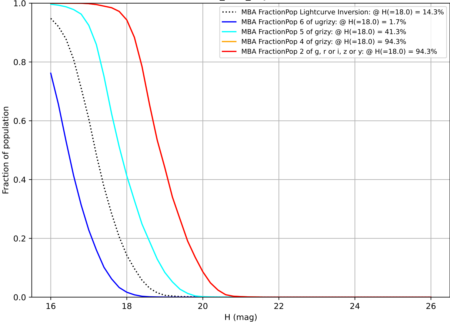
baseline_v4.0_10yrs MBA
