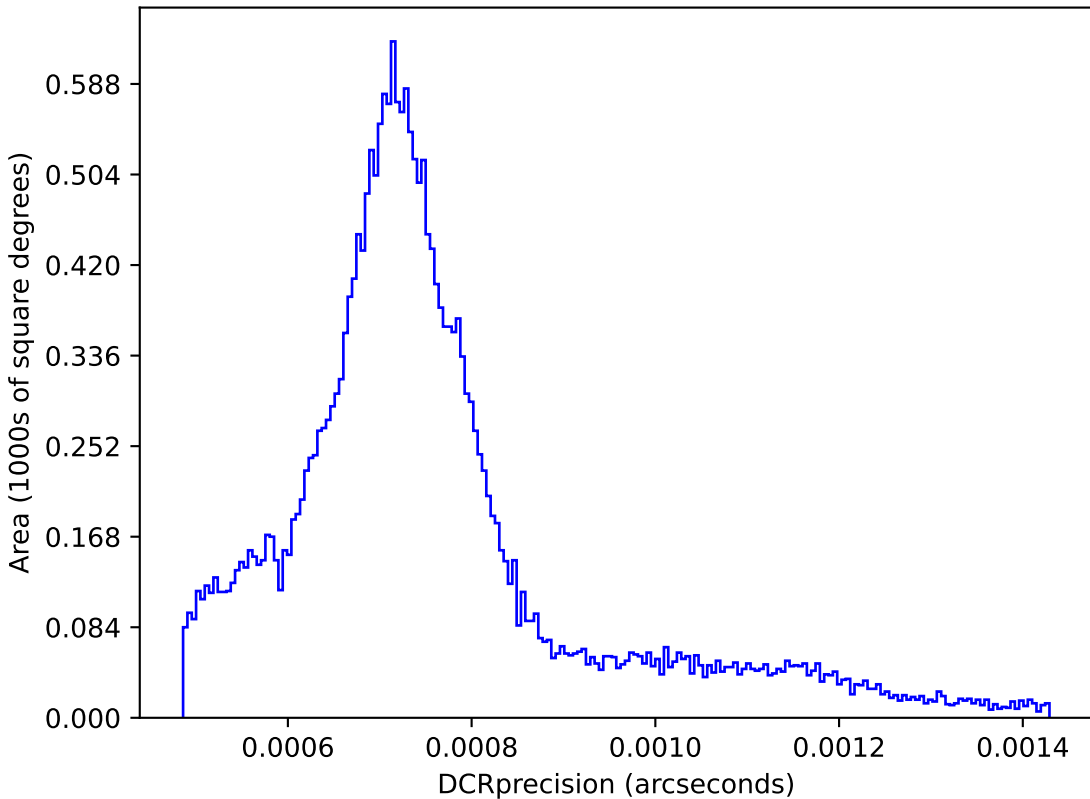
ddf_agn_v3.5_10yrs : DCRprecision
