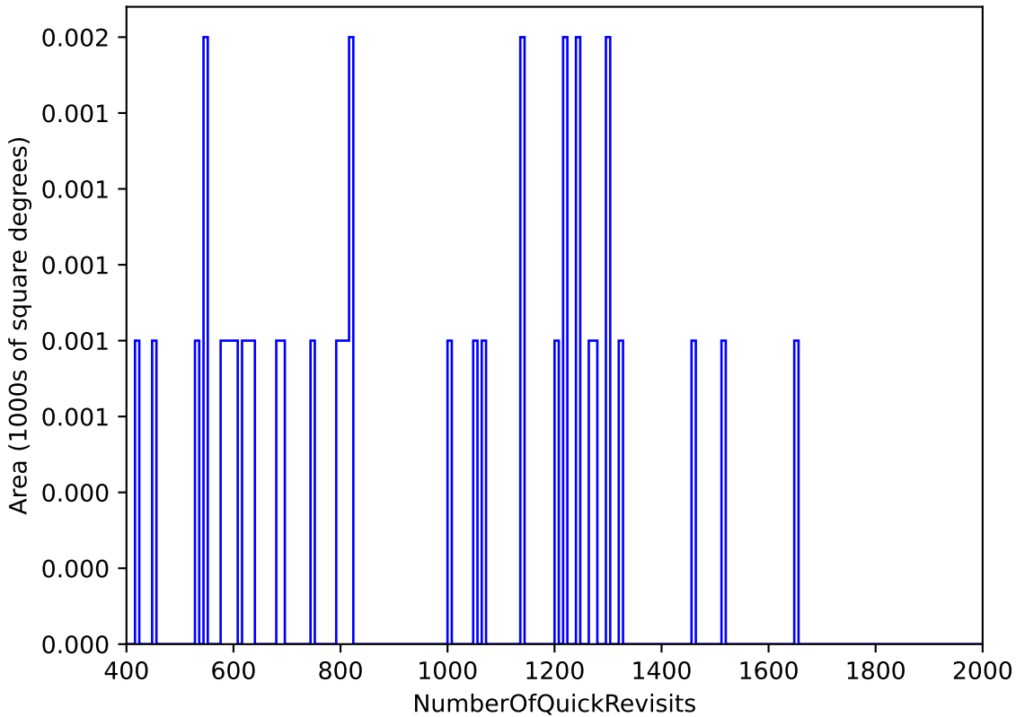
ddf_agn_v3.5_10yrs : NumberOfQuickRevisits
