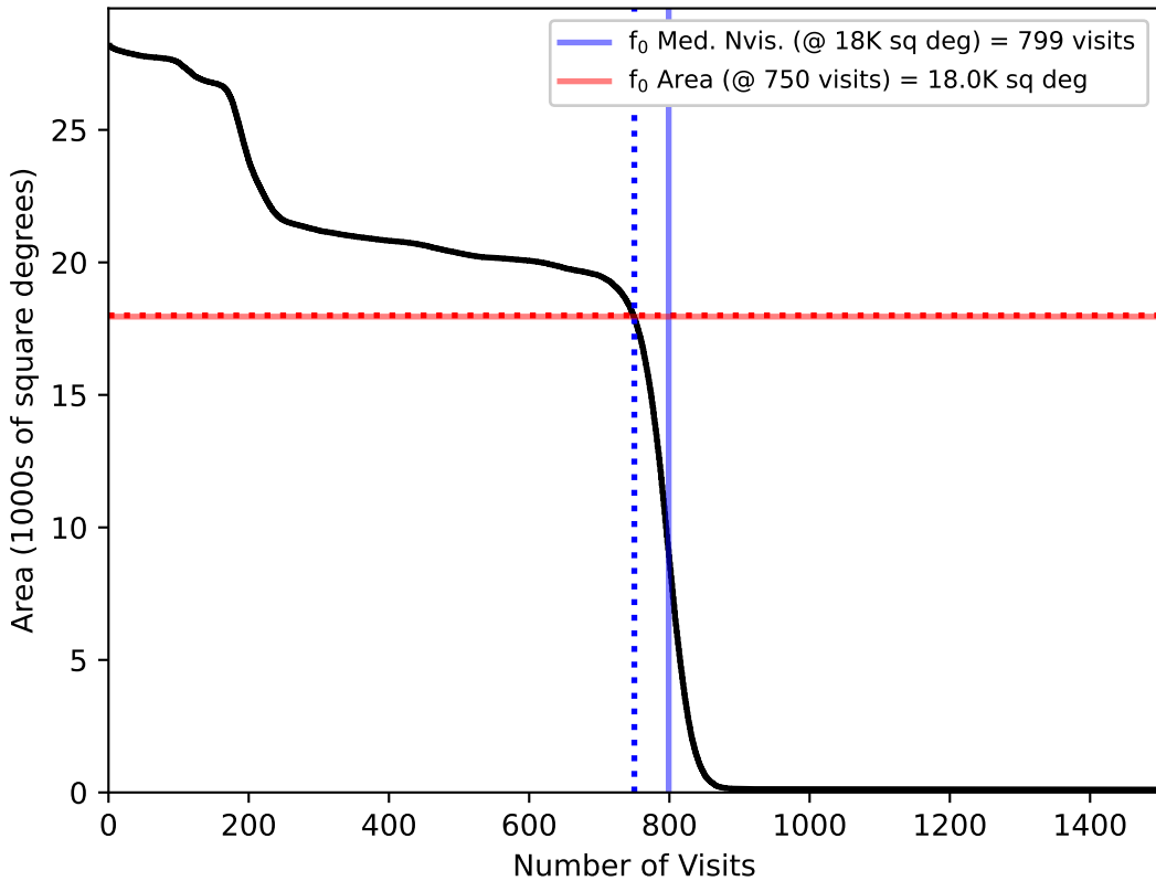
ddf_agn_v3.5_10yrs : f0
