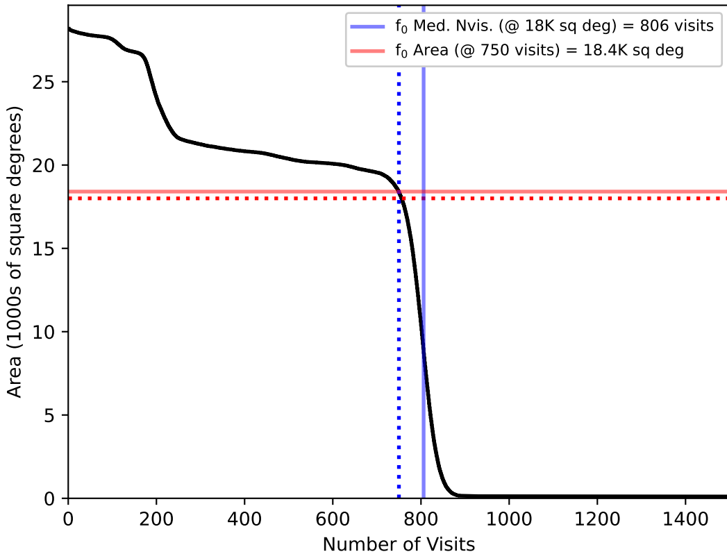
ddf_roll_v3.5_10yrs : fO
